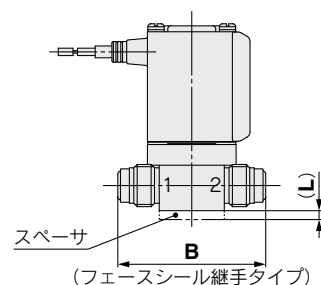
フェースシール継手 コンプレッション継手
