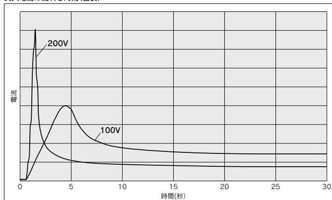
突入電流の流れる時間(目安)
