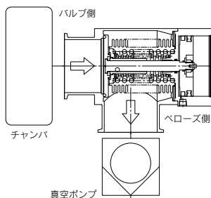
推奨排気方向 [ペロース側に真空ポンプ接続]
