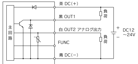
-F PNP (1出力) + アナログ電流出力
