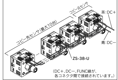
ZS-38-Uを使用した場合の配線例
