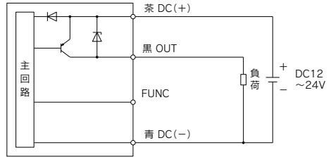
-B PNP (2出力)
