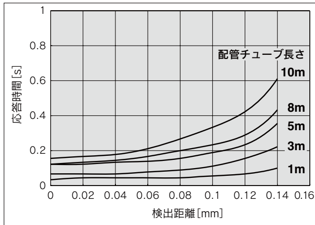
配管チューブ長さ－応答時間
