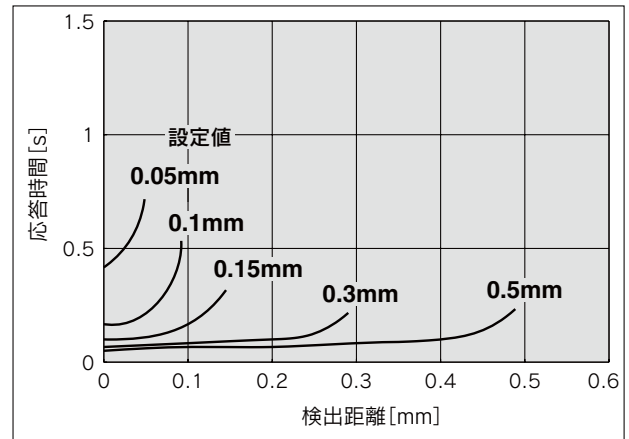
検出距離－応答時間特性
