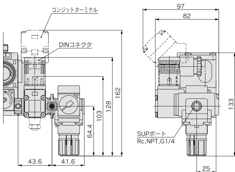
減圧弁+2ポート電磁弁付
