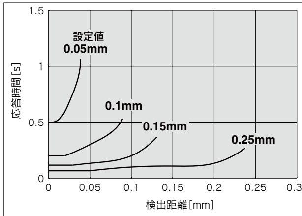
検出距離－応答時間特性
