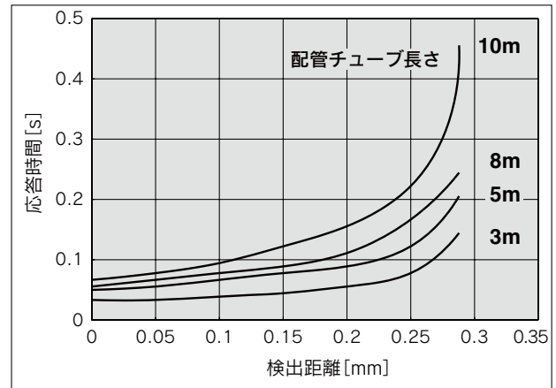
配管チューブ長さ－応答時間
