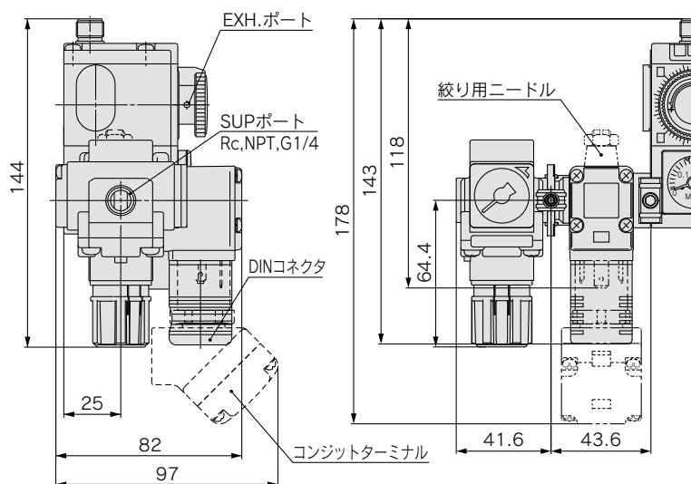
減圧弁+2ポート電磁弁付
