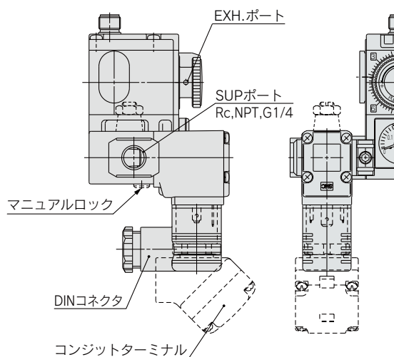
2ポート電磁弁付
