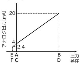
DC4〜20mA
