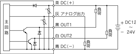
PSE3□3 (T) PNP (2出力) + アナログ電圧出力
