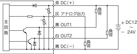
PSE3□2 (T) NPN (2出力) + オートシフト1入力
