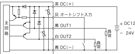
PSE3□5 (T) PNP (2出力) + オートシフト1入力
