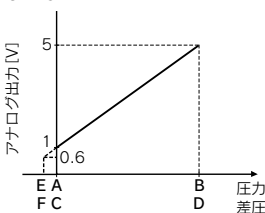
DC1〜5V
