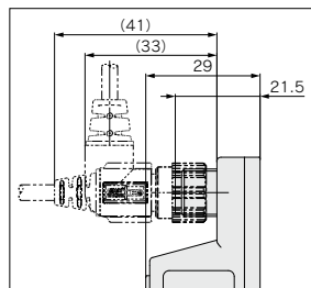
電源・出力接続リード線の場合
