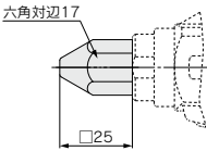
VMG1□-□□-1~04
