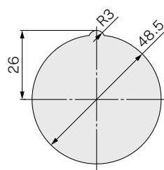
パネルカット寸法 板厚Max.3.5
