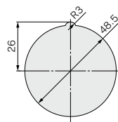
パネルカット寸法 板厚Max.3.5
