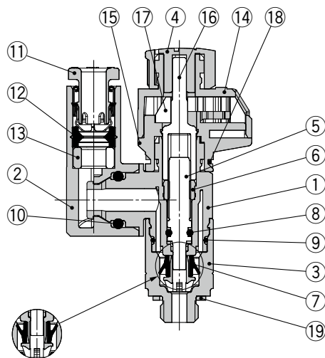
メータイン形 メータアウト形
