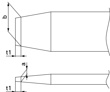
ドライバの先端部形状
