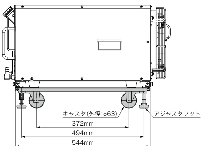
取付状態 (HRR012/018-A-□の場合)
