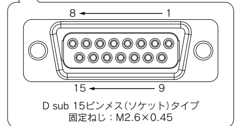
接点入出力信号コネクタ
