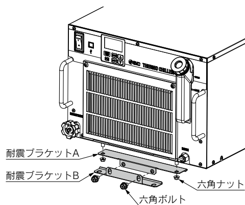
取付完成図
