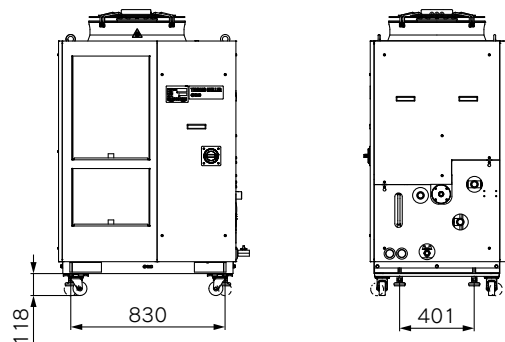
図1 取付状態
