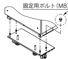
図3 固定用ボルト(8ヶ)
