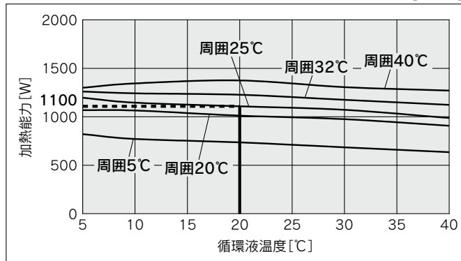
HRS050-A-20 (単相AC200~230V)
