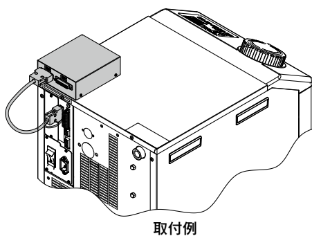
取付例
