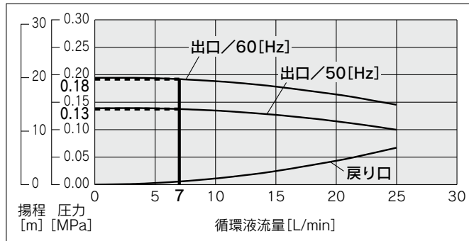
HRS 030 040 -A-W-20 (単相AC200~230V)
