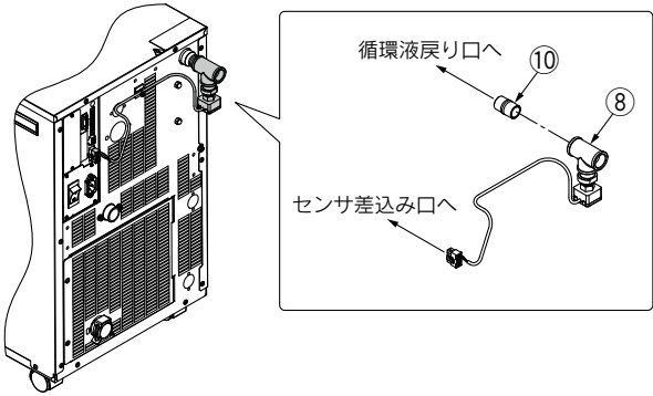
【取付例：HRS012-A-20+HRS-DI009】
