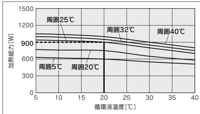
HRS040-A-20 (単相AC200~230V)
