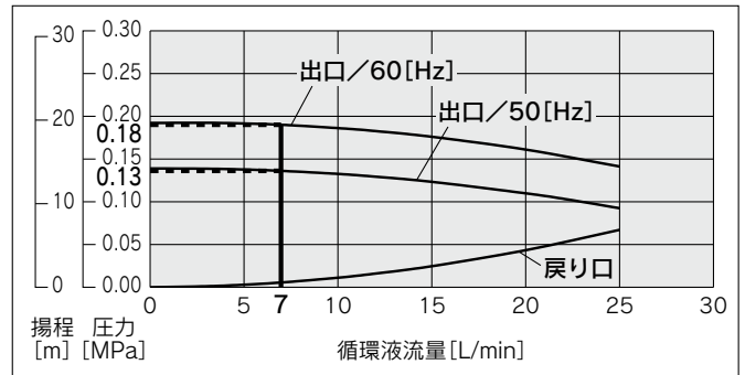
HRS050-A-W-20 (単相AC200~230V)
