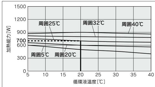
HRS040-W-20 (単相AC200~230V)
