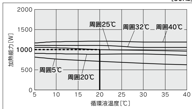
HRS050-W-20 (単相AC200～230V)
