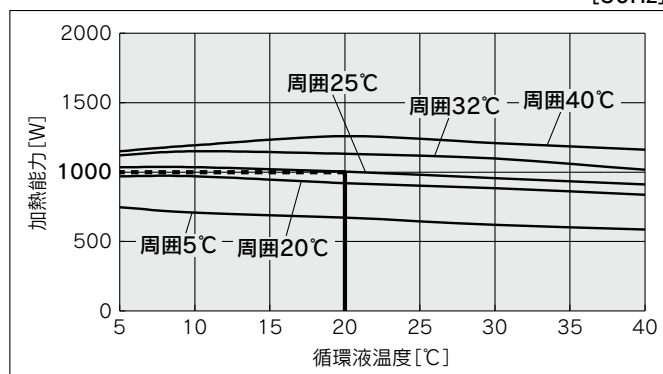
HRS060-A-20 (単相AC200～230V)
