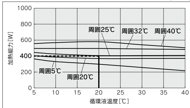
HRS030-W-20 (単相AC200~230V)
