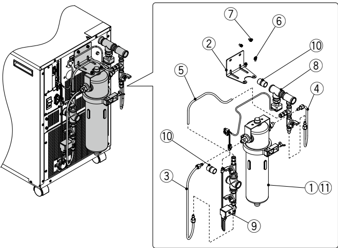
【取付例：HRS012-A-20+HRS-DI009】
