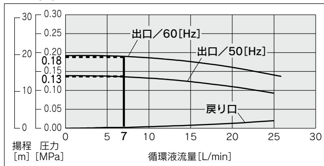
HRS060-A-W-20 (単相AC200~230V)
