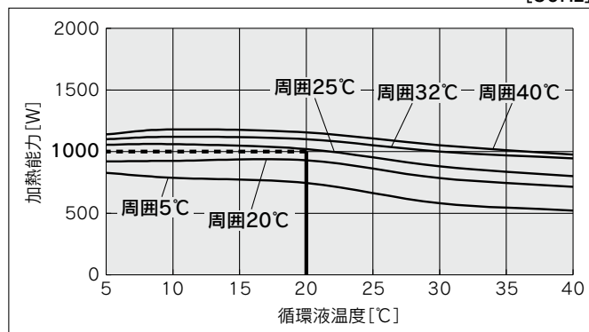
HRS060-W-20 (単相AC200～230V)
